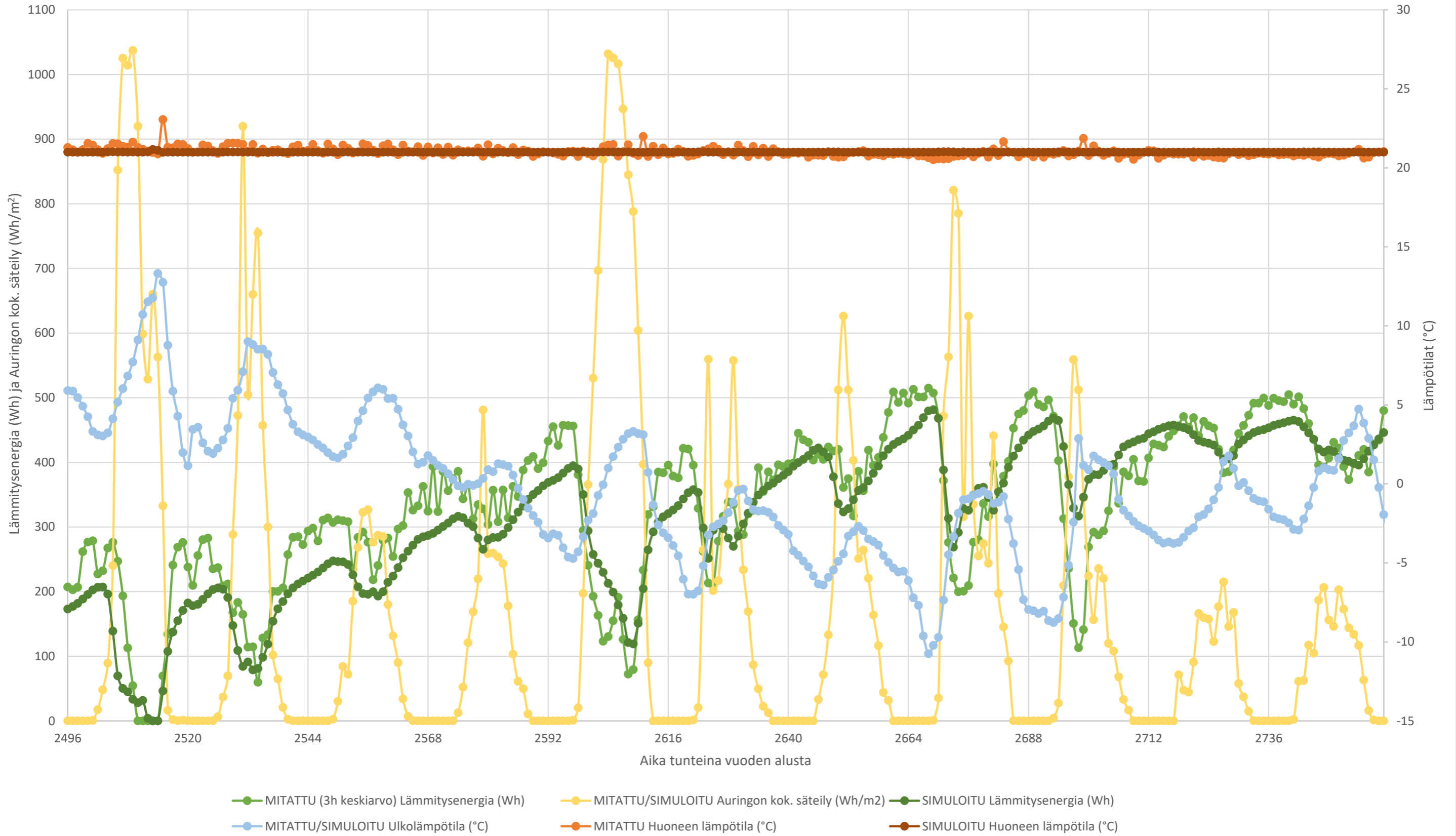
Mitatun ja simuloitun lämmitysenergian kulutuksen vertailu tuntitasolla - Lisäksi käyrästä esitetään mitattu ja simuloitu huonelämpötila, auringon säteilyn määrä sekä ulkolämpötila.
